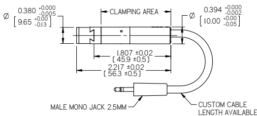
STANDARD MINI LASER
